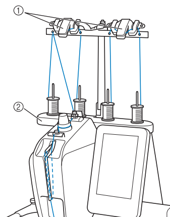
1 Устройство обрезки нити/держатели 2 Подставка для катушек
