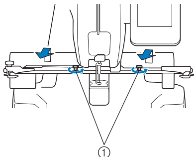
1 Винты с накаткой
