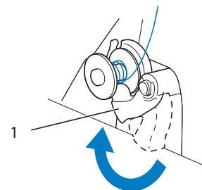
1 Выключатель намотки шпульки
