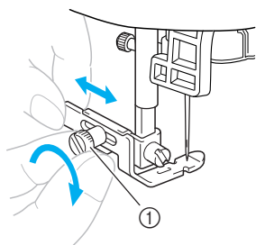
① Стопорный винт
