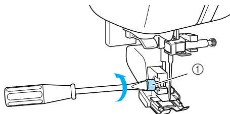
① Винт крепления держателя лапки
