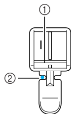
① Стержень на левой стороне лапки ② Точка опускания иглы
